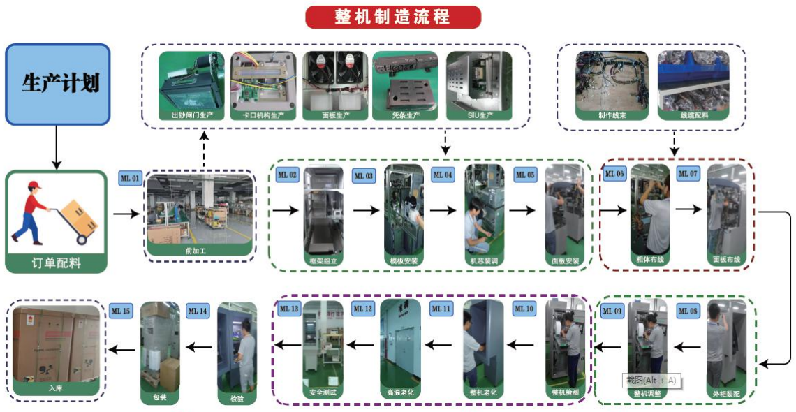
图 2 恒银科技工艺总流程图
